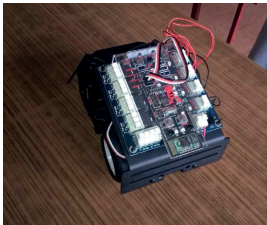
Modeli natjecateljskih robota spasilaca
