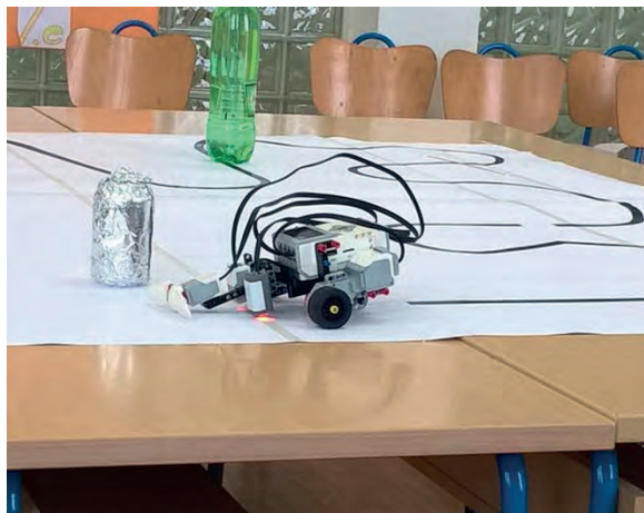
Modeli natjecateljskih robota spasilaca
